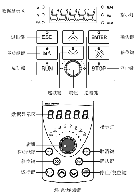
图 4-1 键盘示意图
